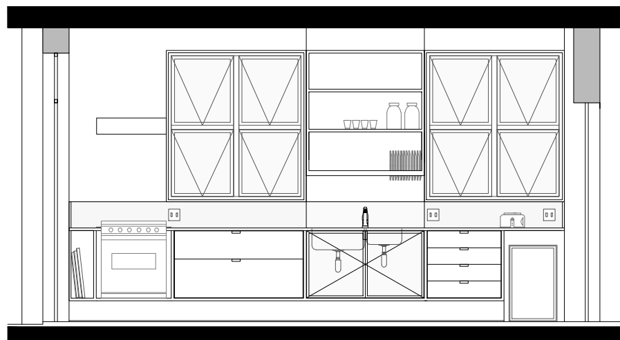
CORTE A ESC.:1:50
