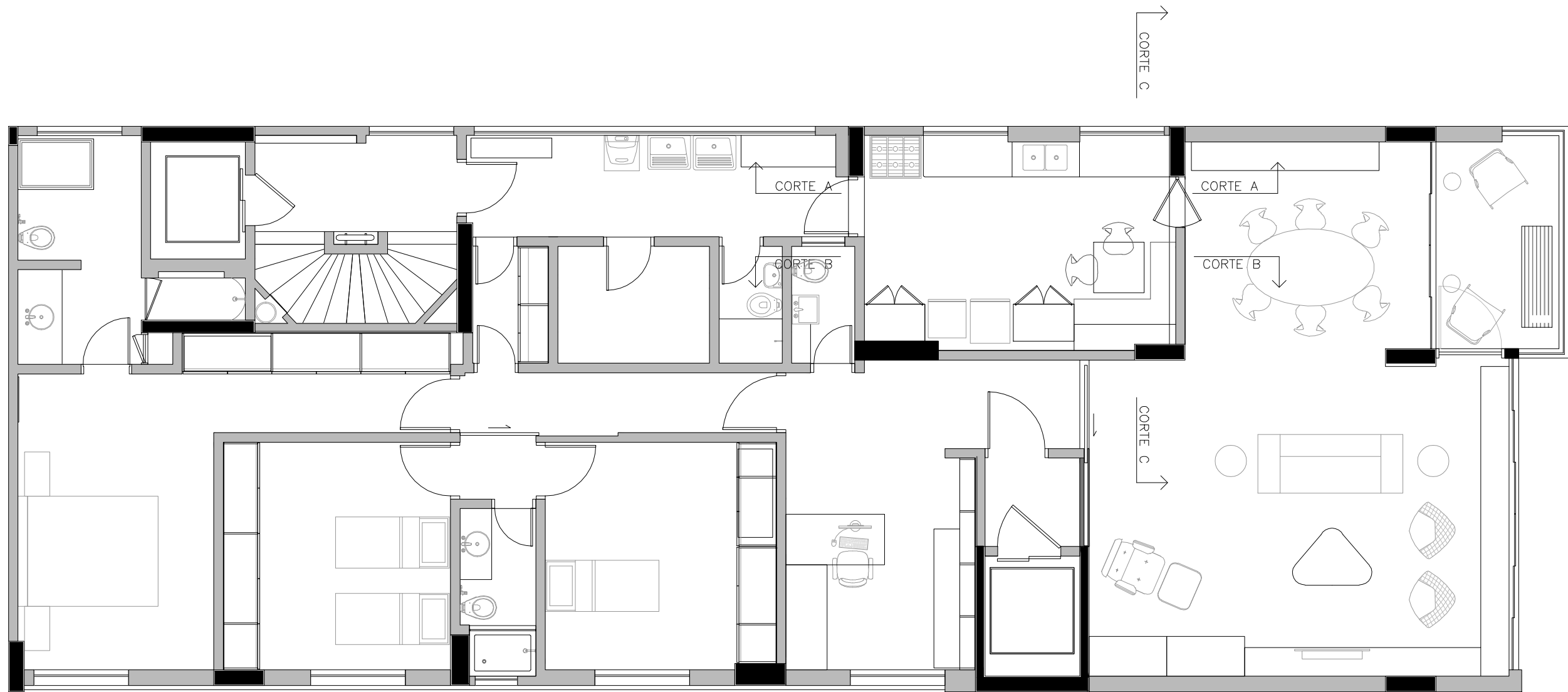
PLANTA ESC. 1:75
