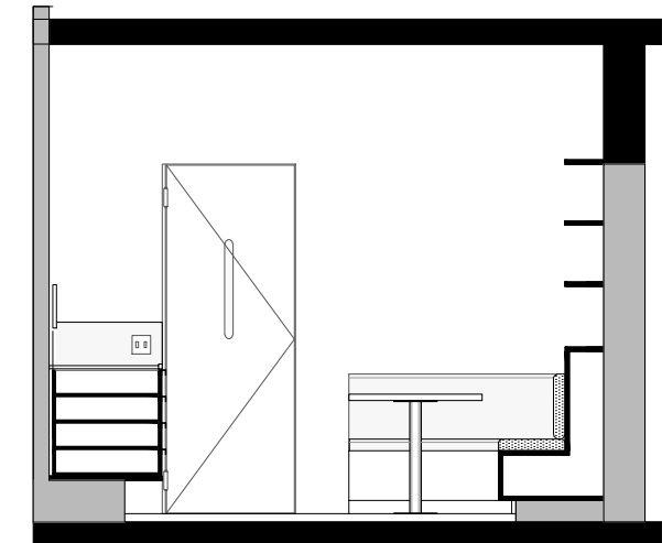
CORTE C ESC.:1:50
