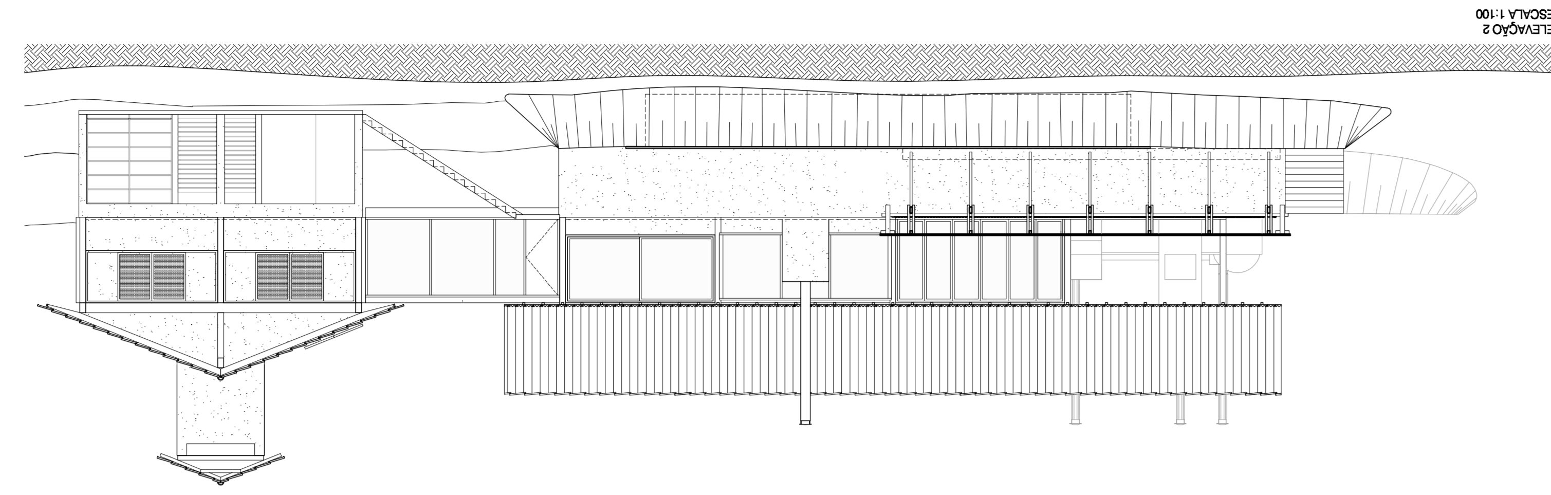
ELEVAÇÃO 2 ESCALA 1:100
